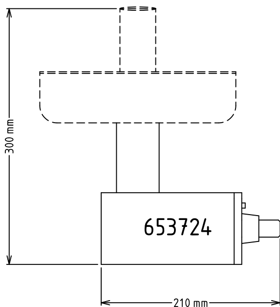
Zij aanzicht
